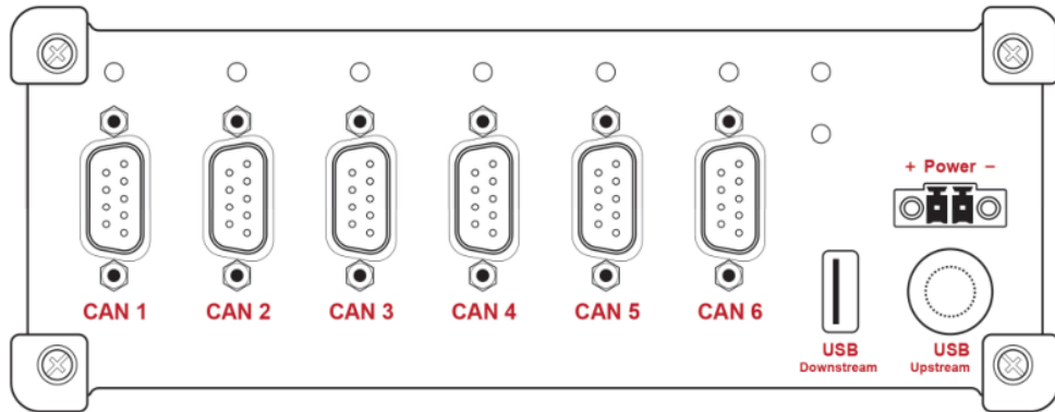
带 D-Sub 接口的 PCAN-USB X6
