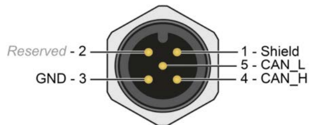
M12 圆形连接器引脚分布
