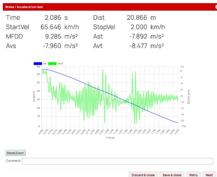
图 1:制动测量示例
