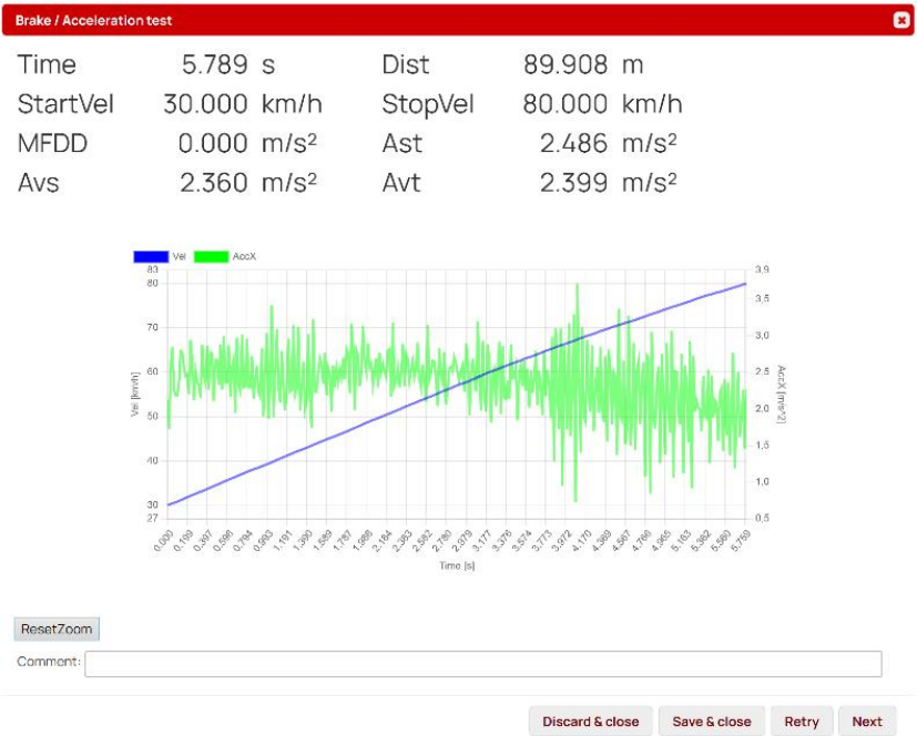
图 2:加速度测量示例
