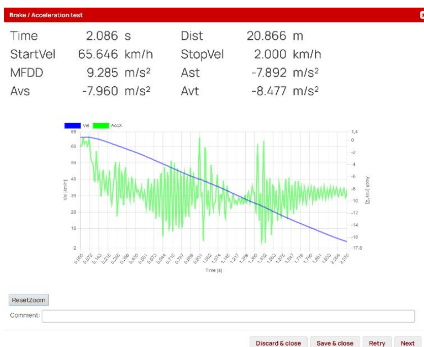
图 1:制动测量示例
