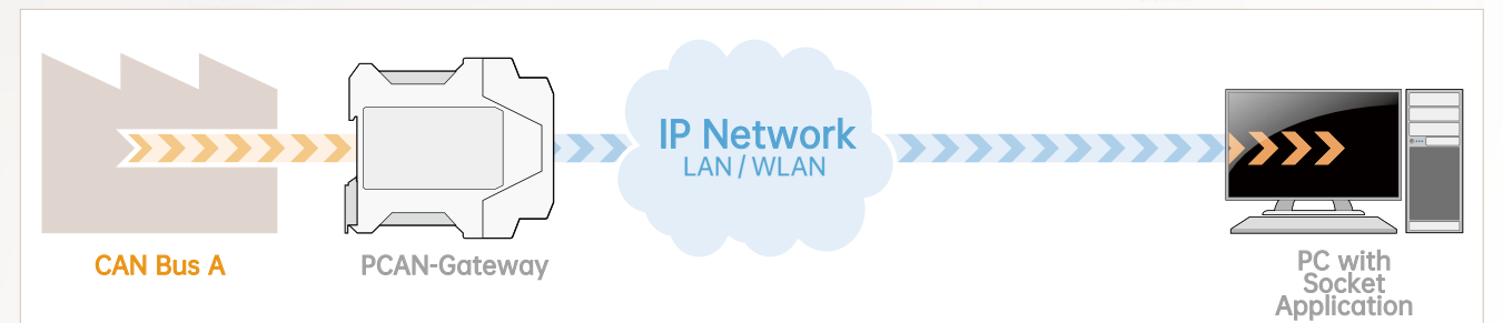
例 3: 经由套接字应用程序连接
